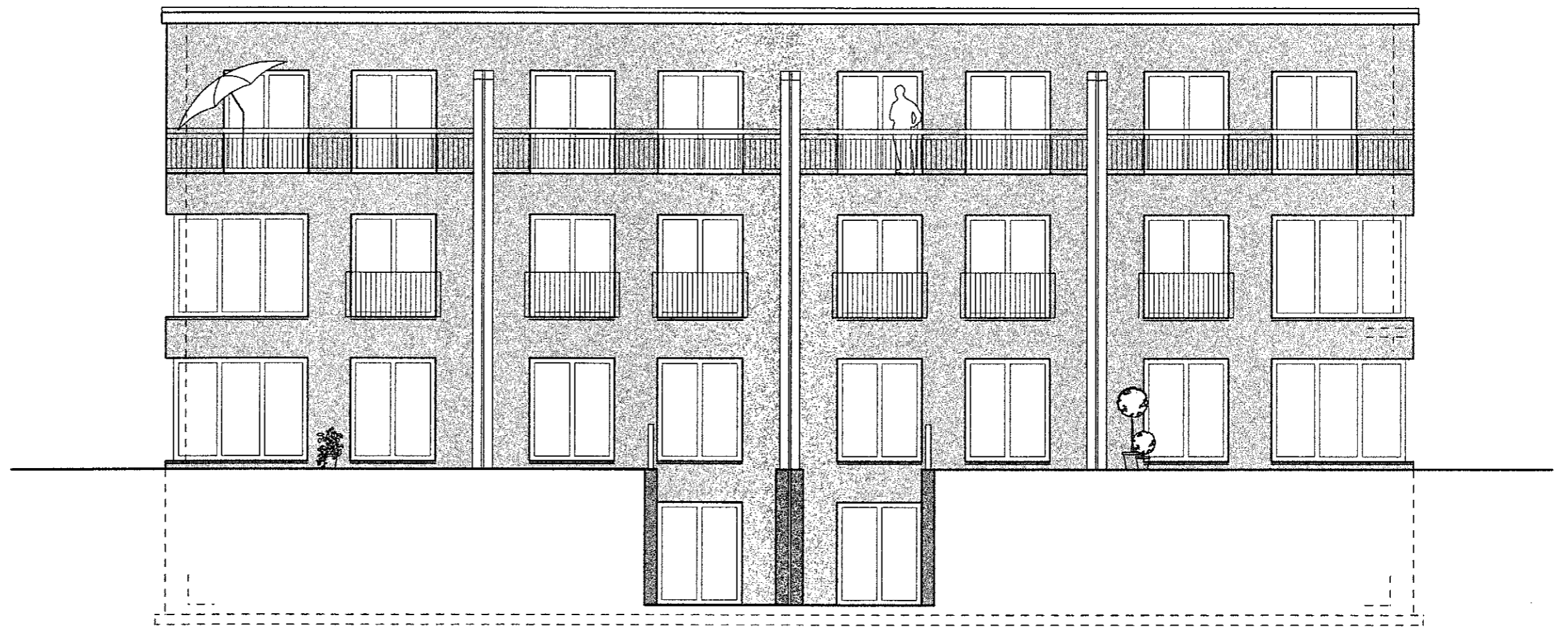
GARTENANSICHT
