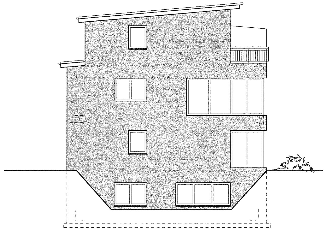
RECHTE SEITENANSICHT
