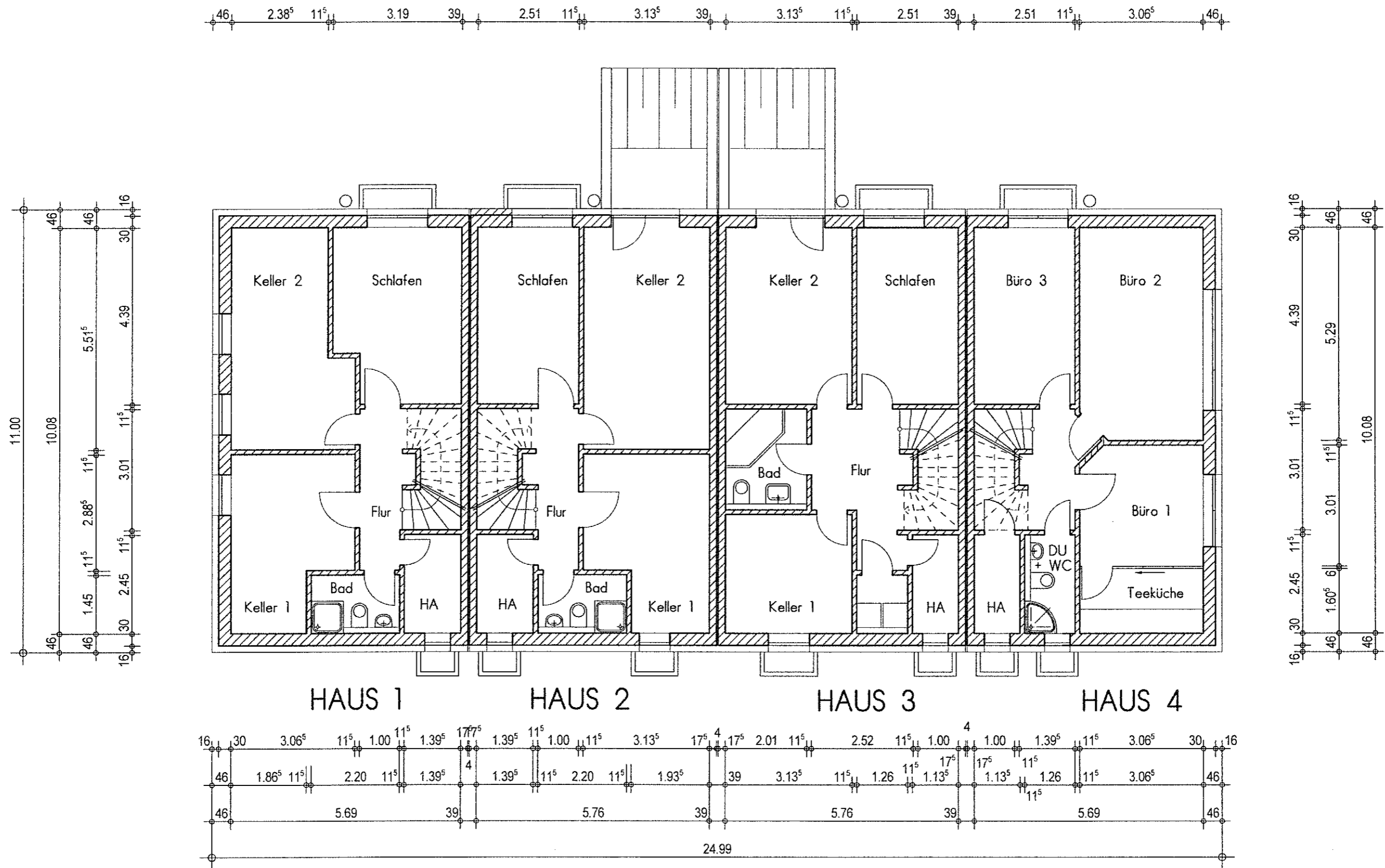
GRUNDRISS KELLERGESCHOSS
