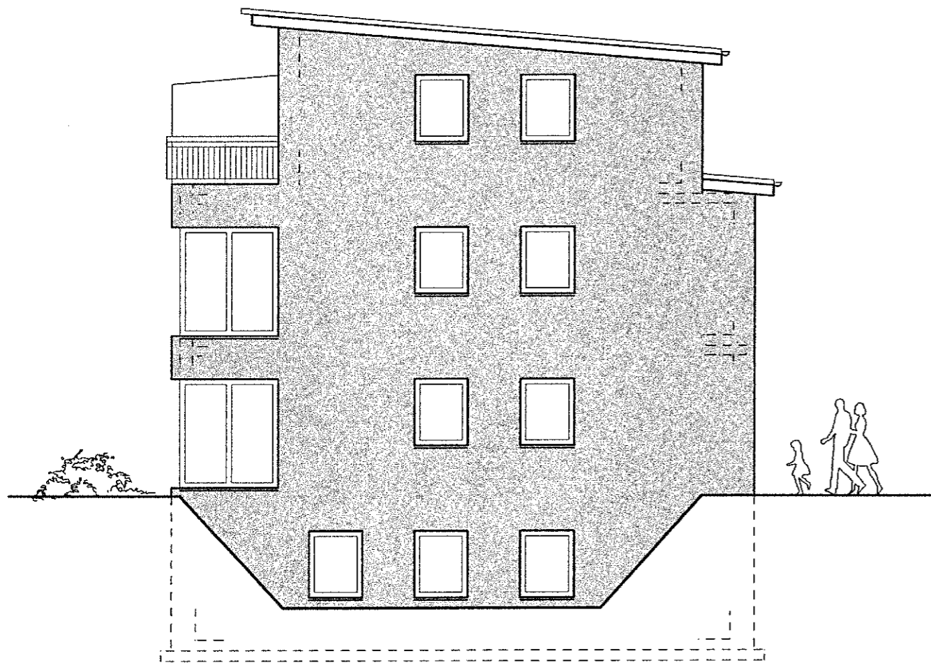
LINKE SEITENANSICHT
